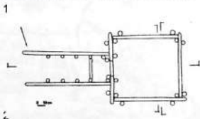
Сактардын жер үстүнө көмүшү: 1 – сырткы көрүнүшү. 2 – схемасы.
